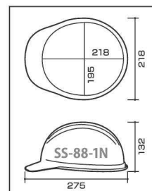
SS-88-1N型寸法図
