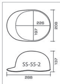
SS-55-2 型寸法図
