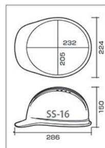
SS-16V 型寸法図
