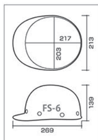
FS-6 型寸法図
