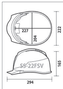
寸法図
