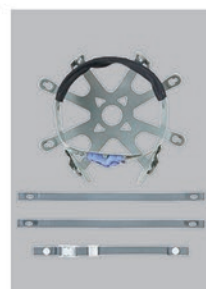
SD 型 - 内装 ・ラチェット式調整 ・耳紐・あご紐付 ▼オープンブライス
