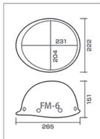
FM-6 型寸法図
