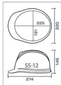
SS-12 型寸法図
