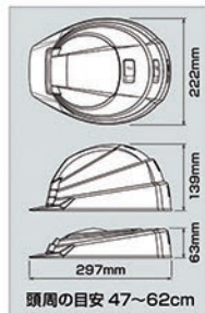
IZANO2 寸法図
