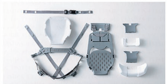
IZANO2-内装
