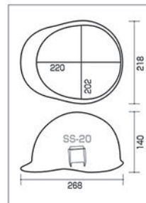
SS-20 型寸法図
