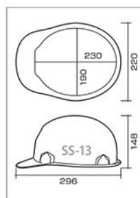
SS-13 型寸法図
