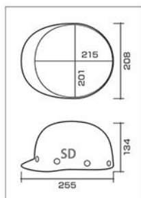
SD 型寸法図
