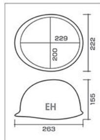
EH型寸法図
