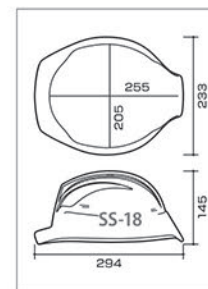
SS-18V 型寸法図
