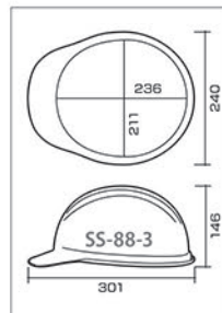
SS-88-3 型寸法図
