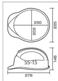
SS-15 型寸法図
