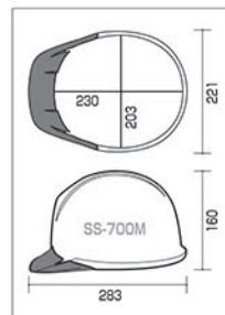
SS-700M 型寸法図
