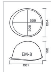
EM-8 型寸法図
