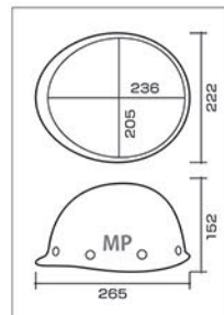
MP 型寸法図
