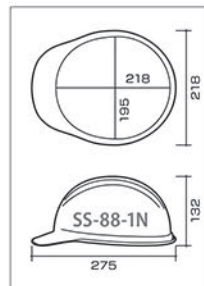
SS-88-1N 型寸法図
