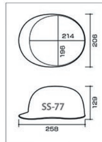
SS-77 型寸法図
