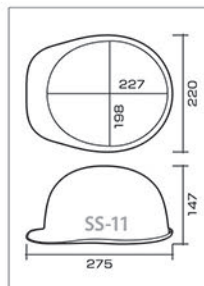
SS-11 型寸法図
